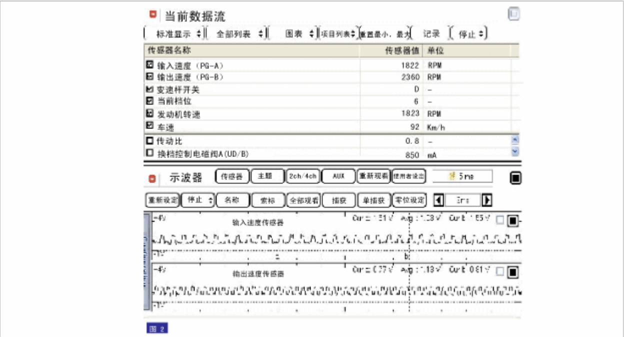
图.1)低速时的输入/输出速度传感器
